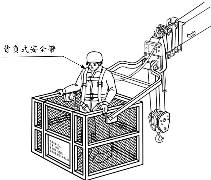
圖 1 起重機吊掛搭乘設備
