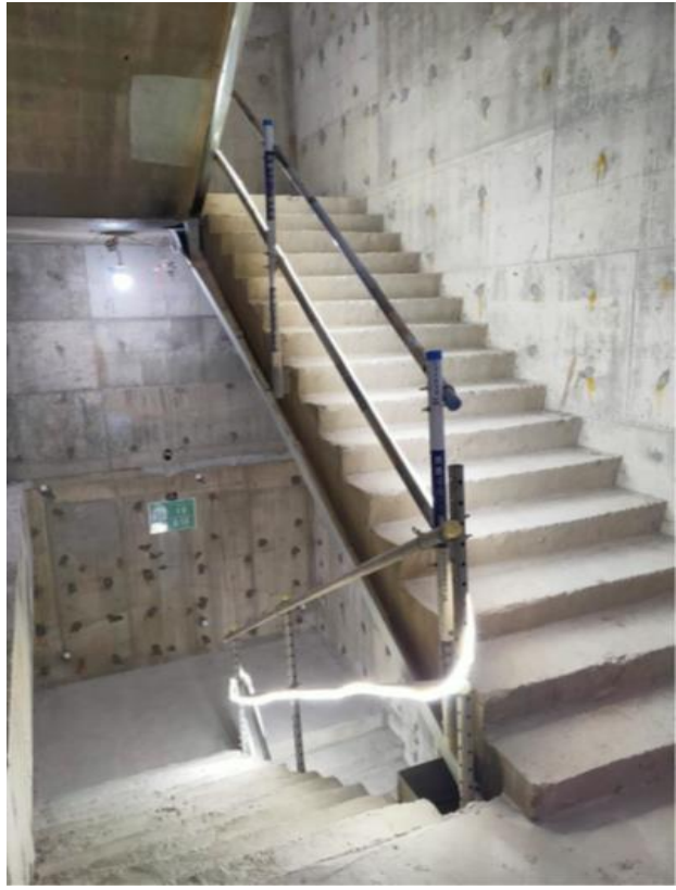
樓梯開口防護，並提供適當照明。
