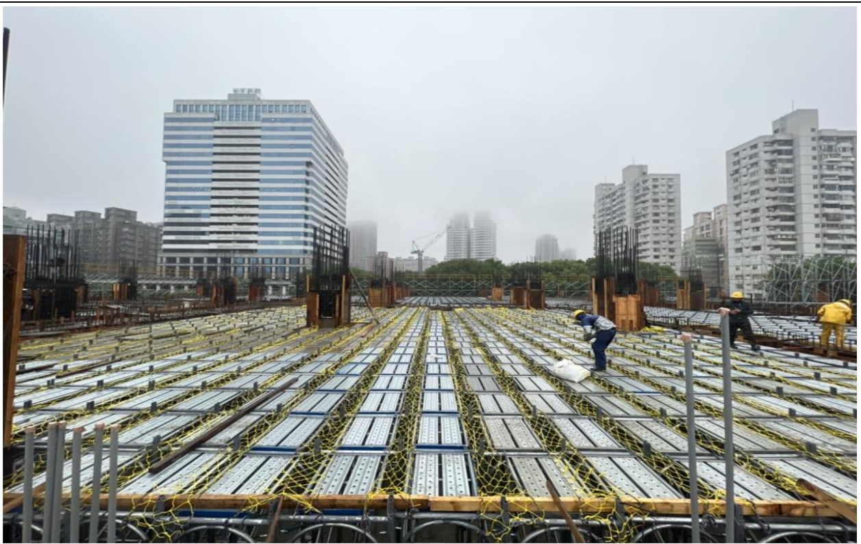
施工排架墜落防護。
