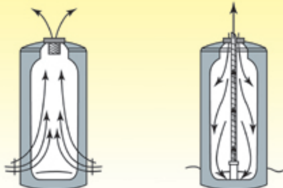
比空氣輕的危害氣體換氣 比空氣重的危害氣體換氣
